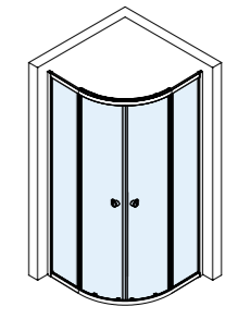
Kwartrond met schuifdeuren 90x90x200 cm (873-888x873-888 mm)
