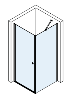
Draaideur met zijwand 90x90x200 cm (873-888x873-888 mm)* 100x100x200 cm (973-988x973-988 mm)
