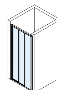
Driedelige schuifdeur 80x200 cm (790-810 mm) 85x200 cm (840-860 mm) 90x200 cm (880-910 mm) 95x200 cm (940-960 mm) 100x200 cm (990-1010 mm)
