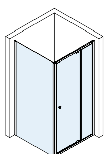
Draaideur met zijwand 90x90x200 cm (830-930x873-888 mm) 100x100x200 cm (930-1030x973-988 mm)
